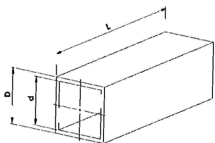
Vierkant/square EN 10305-5
