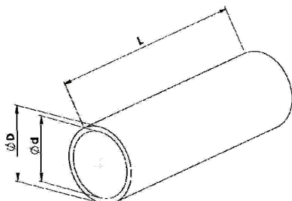
Rund/round EN 10217-7
