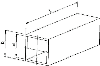
Vierkant/square EN 10305-5
